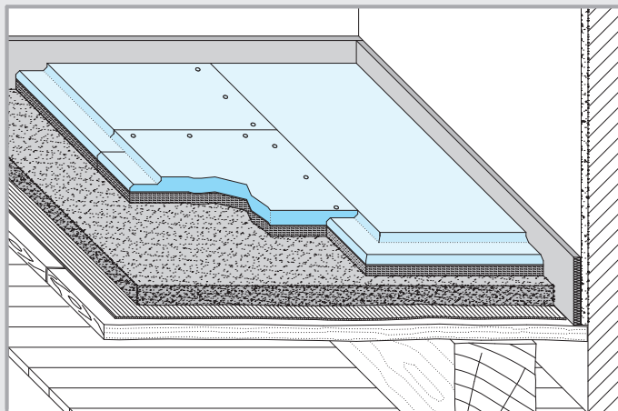
• Ej. F 127.es Knauf Brío elemento compuesto: 18 mm Brío + madera prensada
